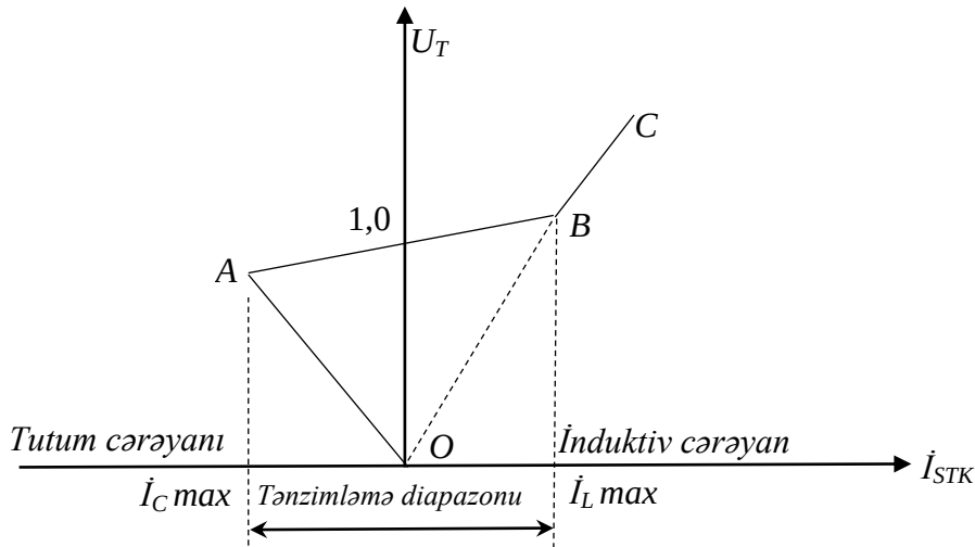
Şəkil 2. STK-nın volt-ampər xarakteristikası
