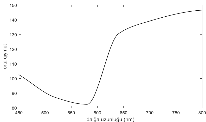
Şəkil 5. Dağ meşə massivinin işığı əksətdirməsinin dalğa uzunluğundan asılılıq qrafiki
