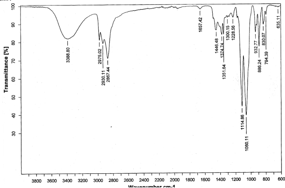
Şək. 1,3-butilenqlikolun n=46,52 olan xloroksipropil efrinin TEA-lı modifikasiının İQ-spektri
