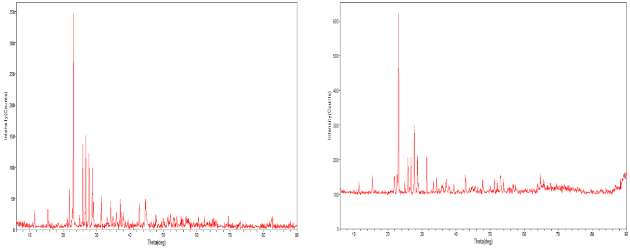
Şəkil 4. a) 20 və b) 60 dövr/dəq rejimlərlə (8 saat) mexaniki qatışdırılmış komponentlərin diffraktoqramları
