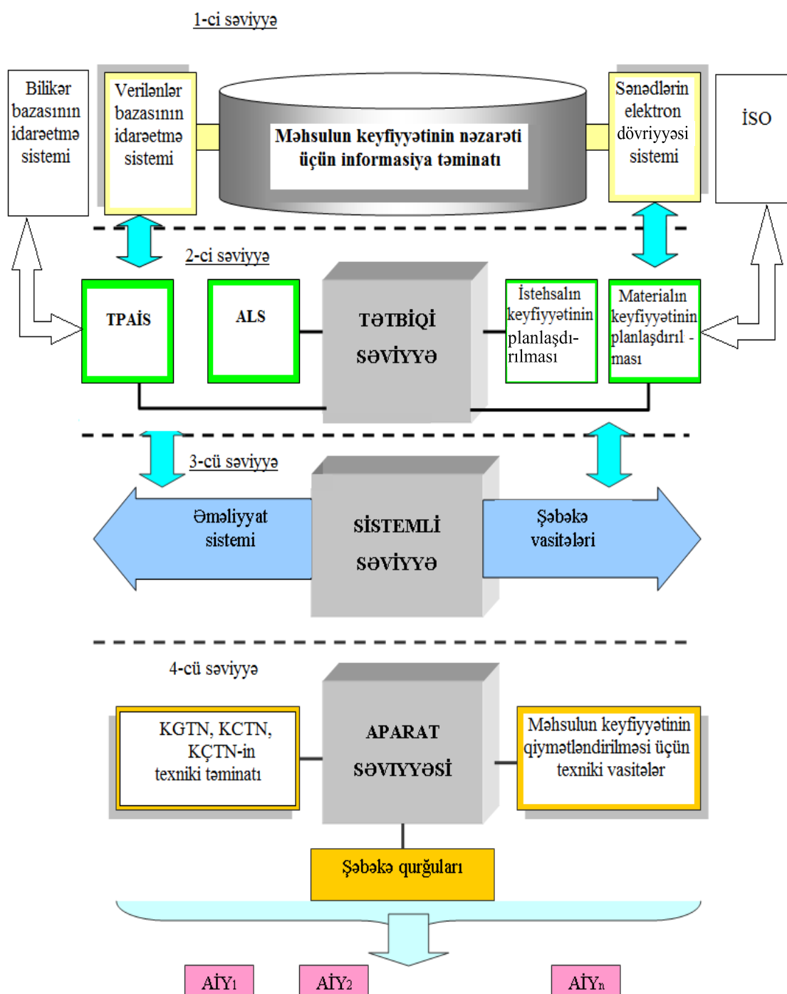
Şəkil 2. Mexaniki yığım istehsalat sexində hazırlanan məhsulun keyfiyyətinə nəzarət sisteminin arxitekturası
