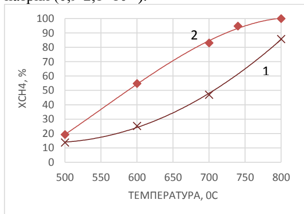
Рис.1. Температурные зависимости степени конверсии метана ( X_{\text{CH}_4} , %) на образцах никелевых катализаторов на основе цеолита типа шабазита от природы катиона цеолита: 1 – K^+ ; 2 – Na^+ .
