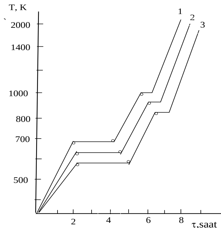
Şəkil 2. Ərintilərin sintez rejimi: 1- As 2 Se 3 , 2- TmAsSe 3 , 3- Tm 2 Se 3
