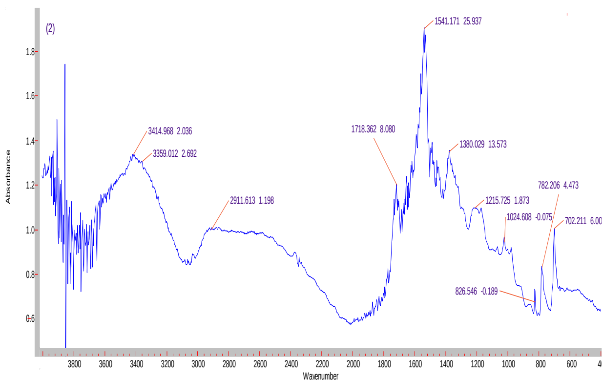
Şəkil 2. 6 fenil 1,3,5 triazin fraqmentli sorbent vanadium (V) ionu ilə əmələ gətirdiyi kompleksin İQ spektri
