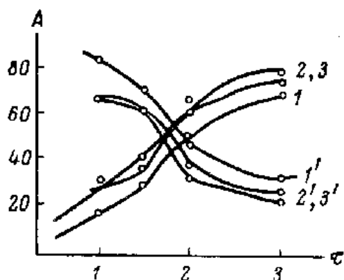
Рис. 3. Влияние продолжительности на выходы диамина (1,2,3) и теломера (1',2',3'). А-выход (%), τ- продолжительность опыта. Соотношение ГА:ЦПД, 1, 1'-1:2; 2,2'-1:2,5; 3,3'-1:3.
