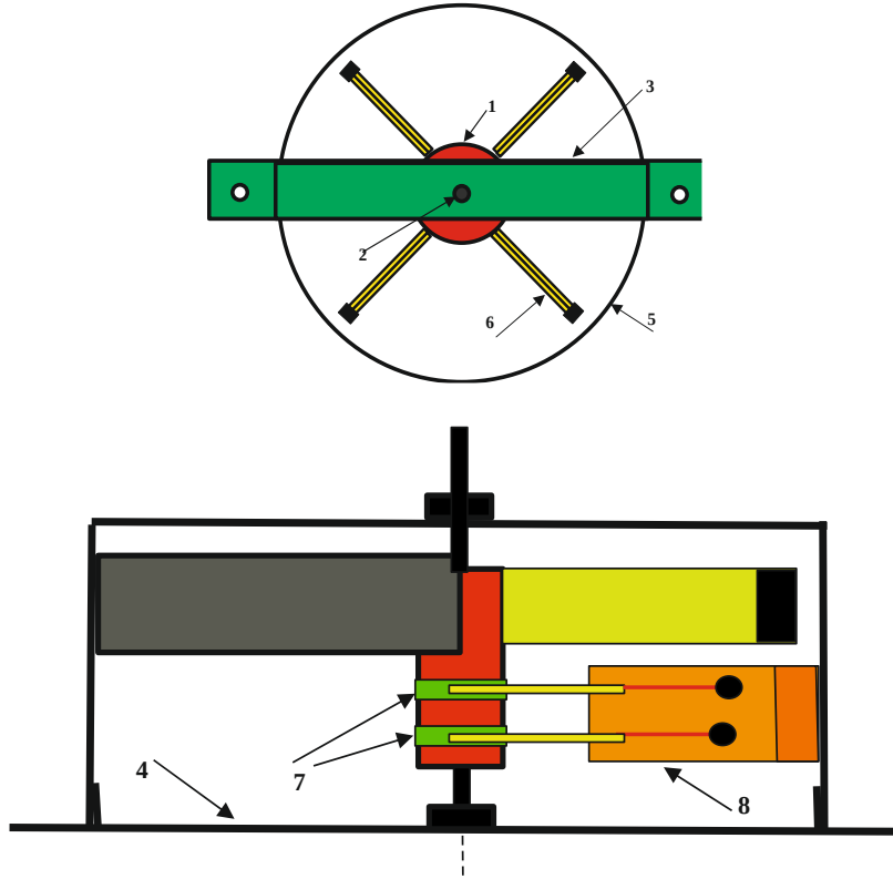
Şəkil. Ətalətli pyezoelektrik addım mühərriki.
