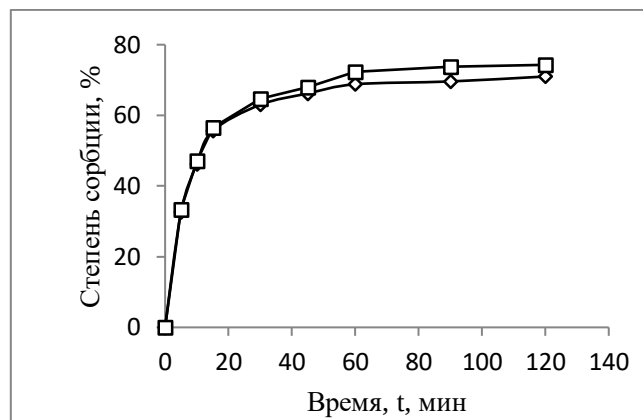
Рис. 3. Зависимость степени сорбции от времени контакта для сорбентов МК-Дц-Ст-Na и МК-Дц-Ст-NH 4 , C_0=0.32 \text{ г л}^{-1} , масса сорбента 1.25 \text{ г л}^{-1} , V = 0.04 \text{ л} , 20^\circ\text{C} )
