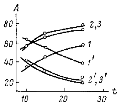
Рис. 4. Влияние температуры при ( \text{TiCl}_4 15 мол.% и продолжительности 3 часа) на выходы диамина и теломера А-выход (%), t-температура ( ^{\circ}\text{C} ). (час). Соотношение ГА:ЦПД, 1, 1'-1:2; 2,2'-1:2,5; 3,3'-1:3.
