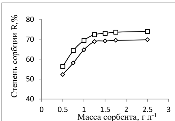
Рис.2. Графики зависимости степени сорбции от массы сорбента для сорбентов МК-Дц-Ст-Na и МК-Дц-Ст-NH 4 . C_0 = 0.32 \text{ г л}^{-1} ( 0.005 \text{ моль л}^{-1} ), V = 0.04 \text{ л} , 60 \text{ мин} , 20^\circ\text{C}
