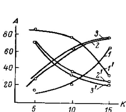
Рис. 1. Влияние количества \text{TiCl}_4 , \text{TiCl}_4 , K (мол. % на взятый ГА) на выходы диамина А (%) от теоретически возможного (в (1,2,3) расчете на взятый \text{TiCl}_4 ). 1,2,3-при температуре 20° и продолжительности 3 часа. Соотношение ГА, ЦПД: 1,1'- 1:2, 2,2'-1:2.5, 3,3'-1:3
